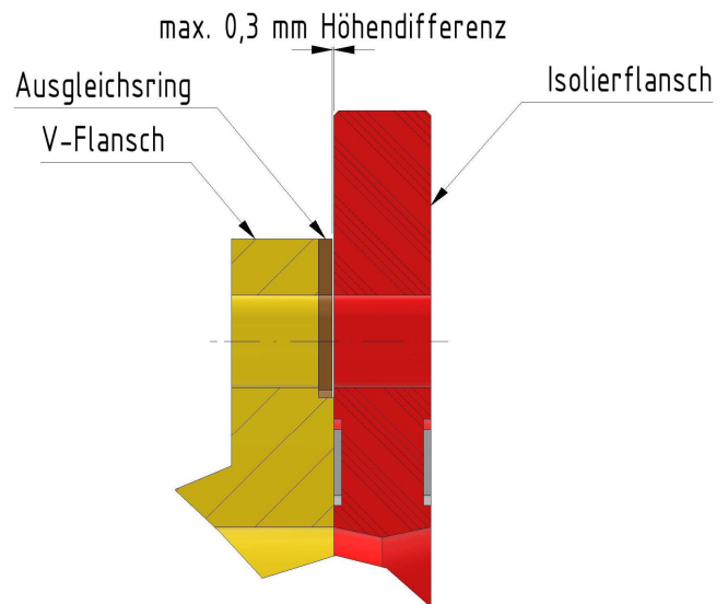
Abbildung 7: Ausgleichringmontage
