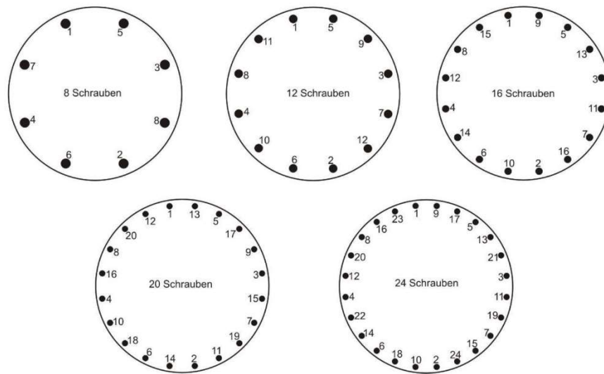
Abbildung 2: Anzugsreihenfolge der Schraubenbolzen
