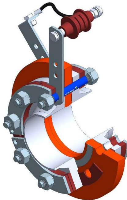
Abbildung 1: Montagebeispiel mit Kabellasse und Funkenstrecke
